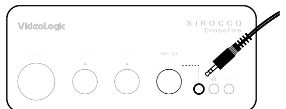
Abbildung 4: Stereo-Audiogeräte an Eingang 3 anschließen
